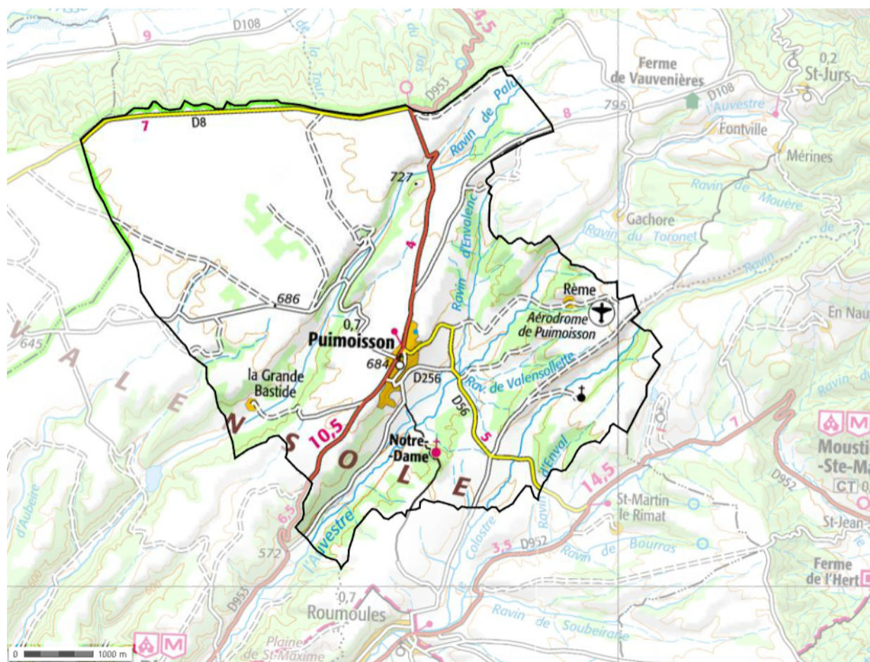
Illustration 3 : Situation de la commune de Puimisson sur fond topographique (source : géoportail.fr)
