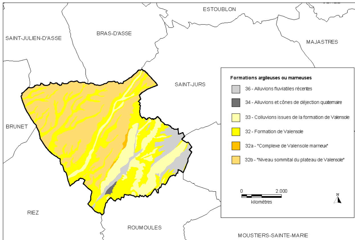
Illustration 5 : Extrait de la carte synthétique des formations argileuses et marneuses couvrant la commune de Puimoisson
