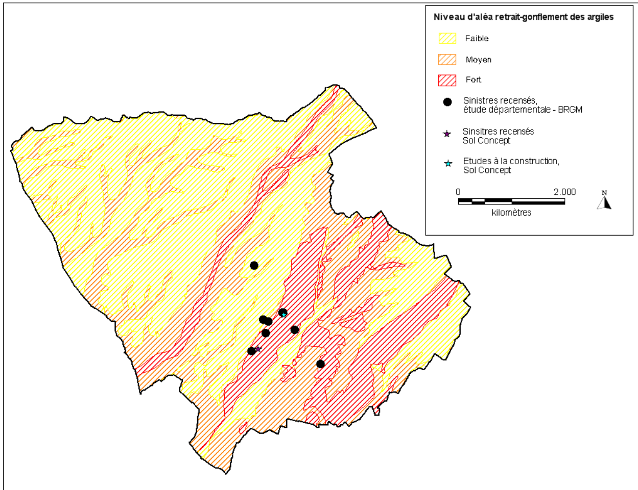
Illustration 7 : Carte d'aléa retrait-gonflement des argiles sur la commune de Puimoisson
