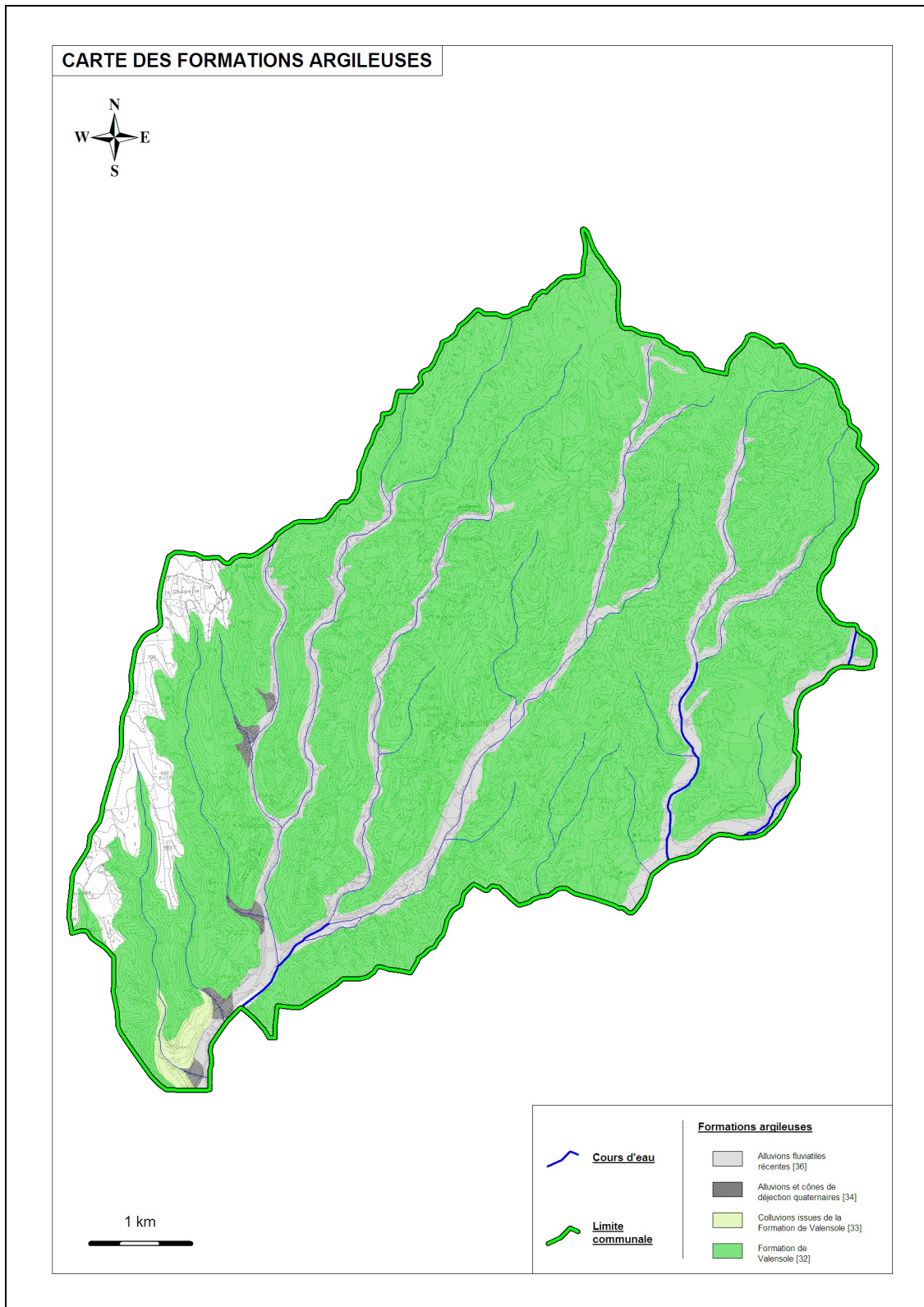
Figure 11 : Carte synthétique des formations argileuses ou marneuses
