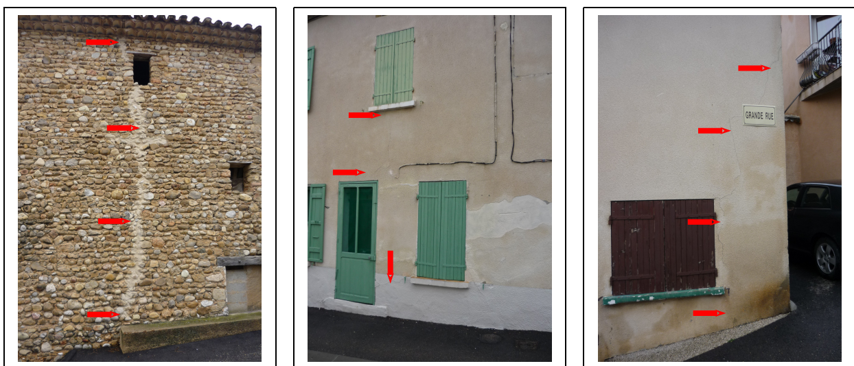
Figure 12 : Fissures sur des maisons (Grande Rue) [Source : IMS RM ]
