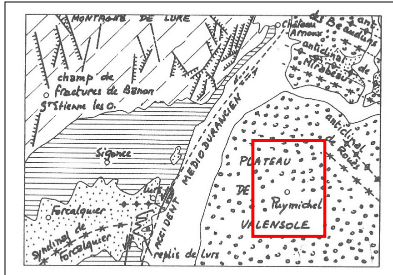
Figure 4 : Cadre géologique du Plateau de Valensole et localisation de la zone d'étude
