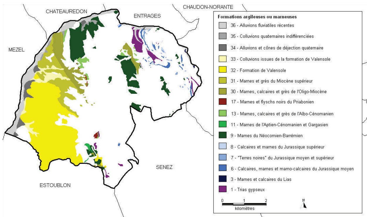
Illustration 5 : Extrait de la carte synthétique des formations argileuses et marneuses couvrant la commune de Beynes
