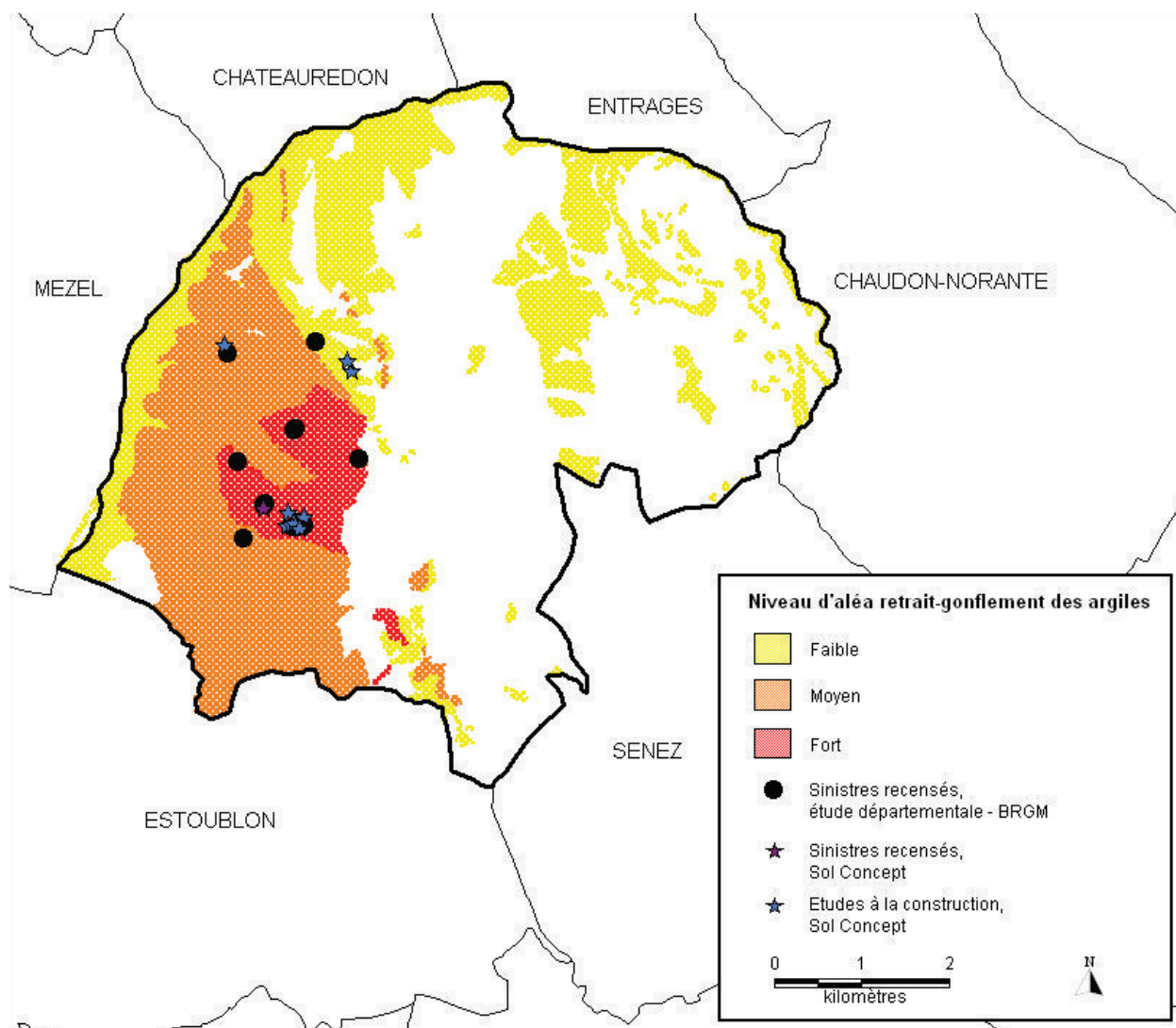
Illustration 7 : Carte d'aléa retrait-gonflement des argiles sur la commune de Beynes
