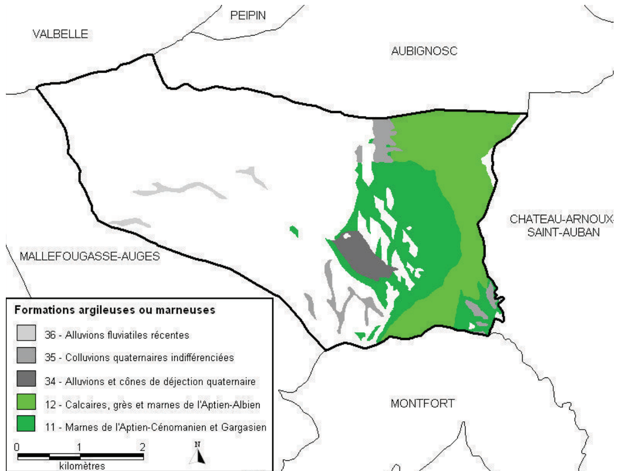
Illustration 5 : Extrait de la carte synthétique des formations argileuses et marneuses couvrant la commune de Châteauneuf Val Saint Donat
