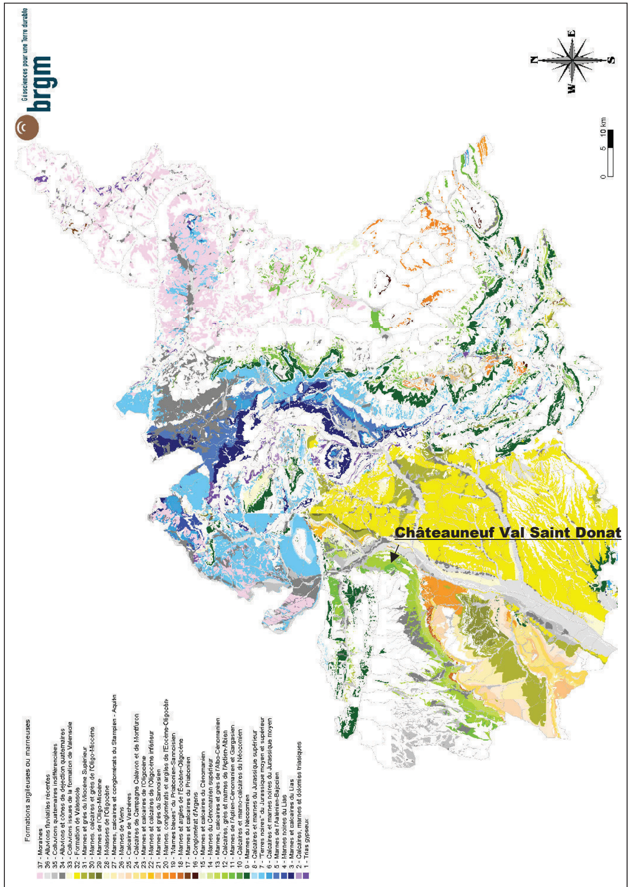
Illustration 4 : Situation de la commune de Châteauneuf Val Saint Donat sur la carte synthétique des formations argileuses et marneuses du département des Alpes-de-Haute-Provence
