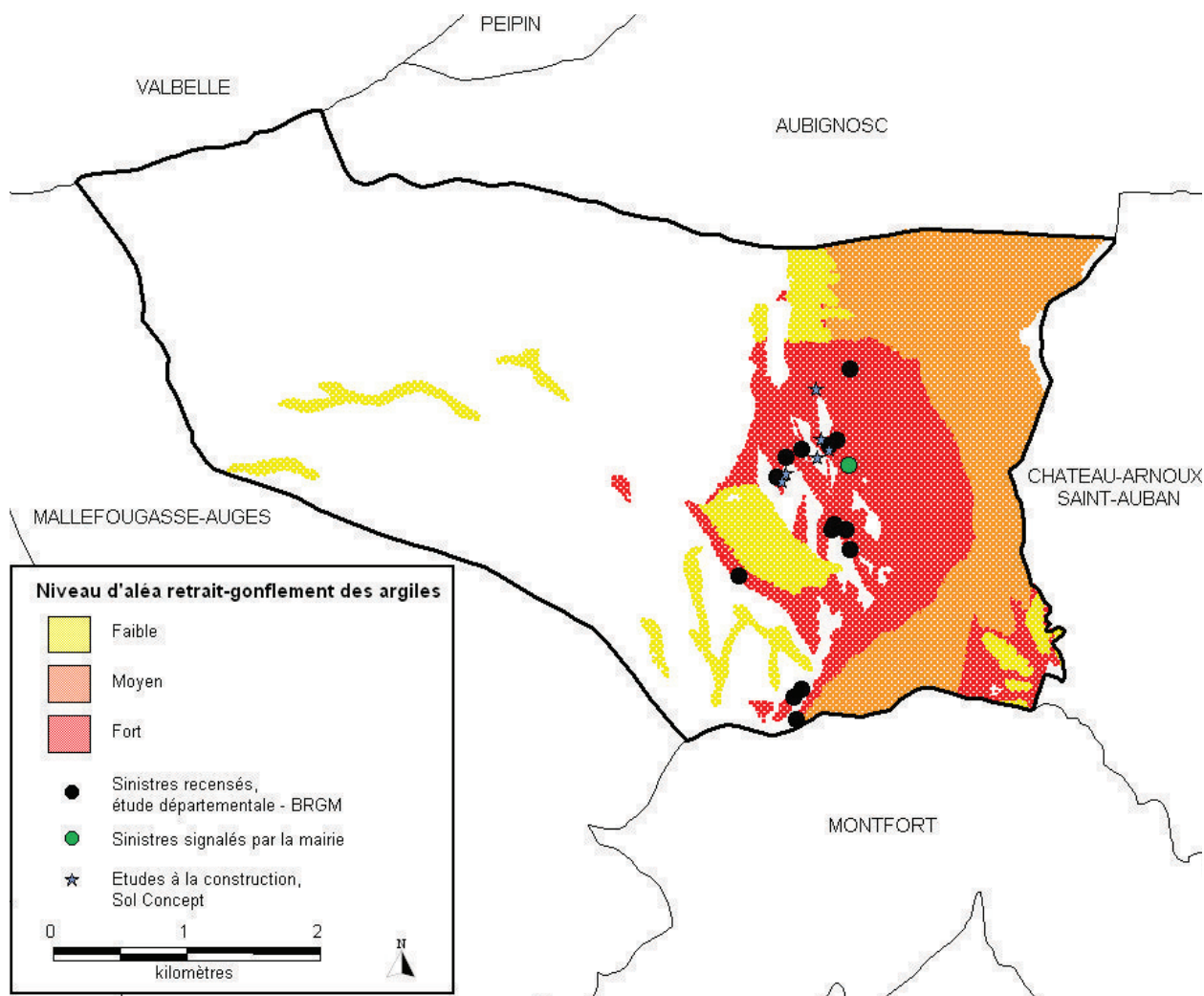
Illustration 7 : Carte d'aléa retrait-gonflement des argiles sur la commune de Châteauneuf Val Saint Donat
